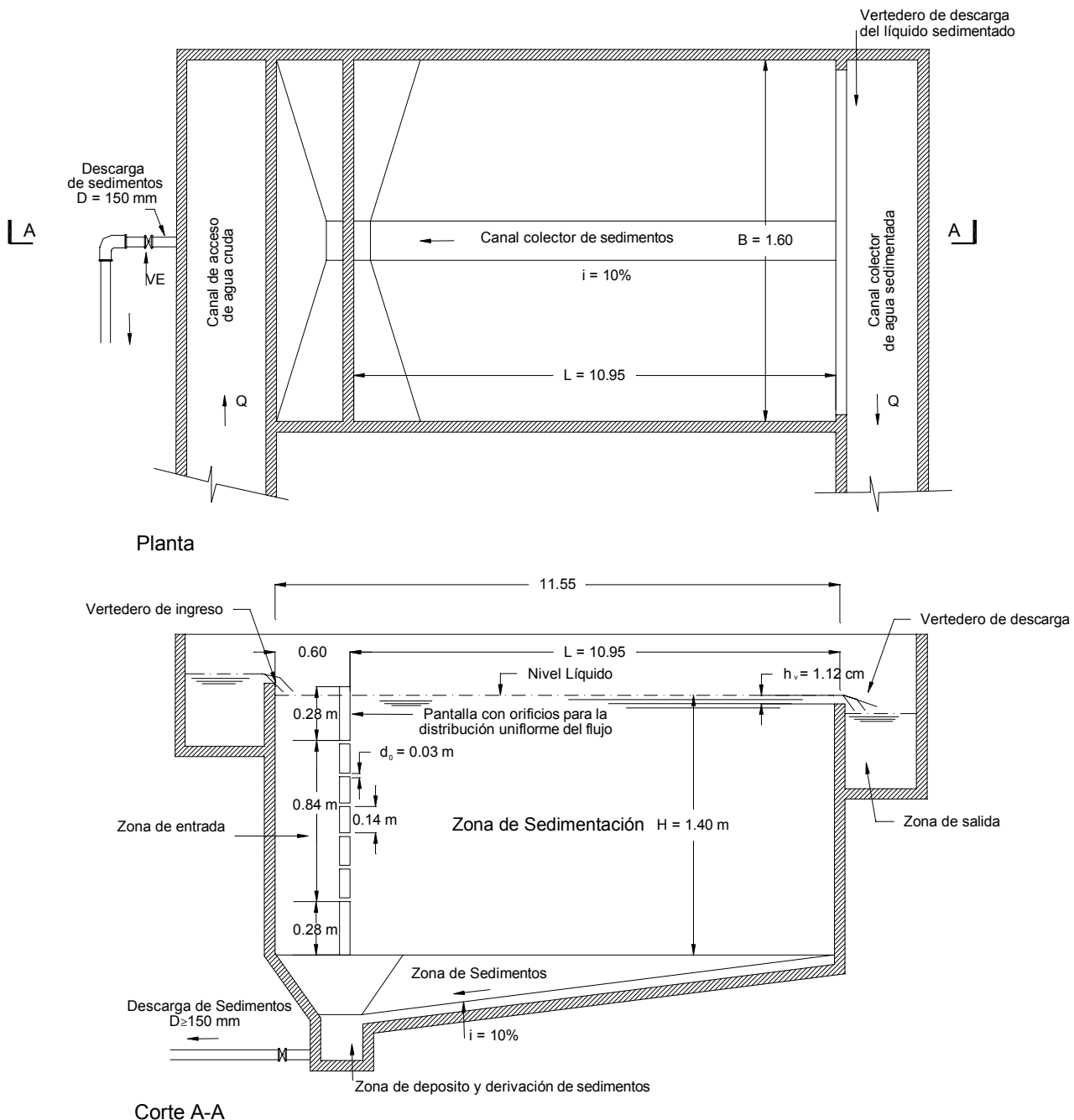
Figura 4. Sedimentador simple
